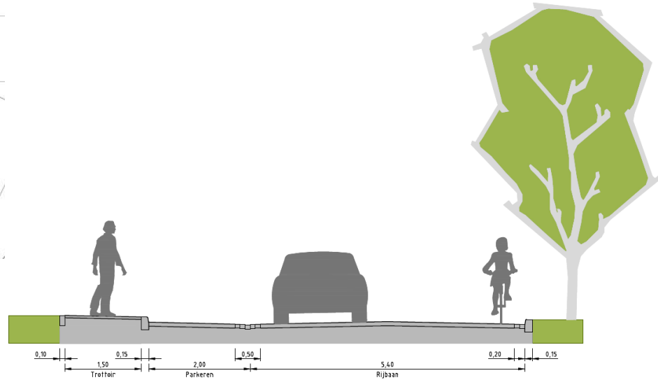
Principe profiel Schaal 1:50
